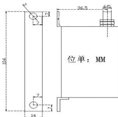
图一 模块尺寸图
