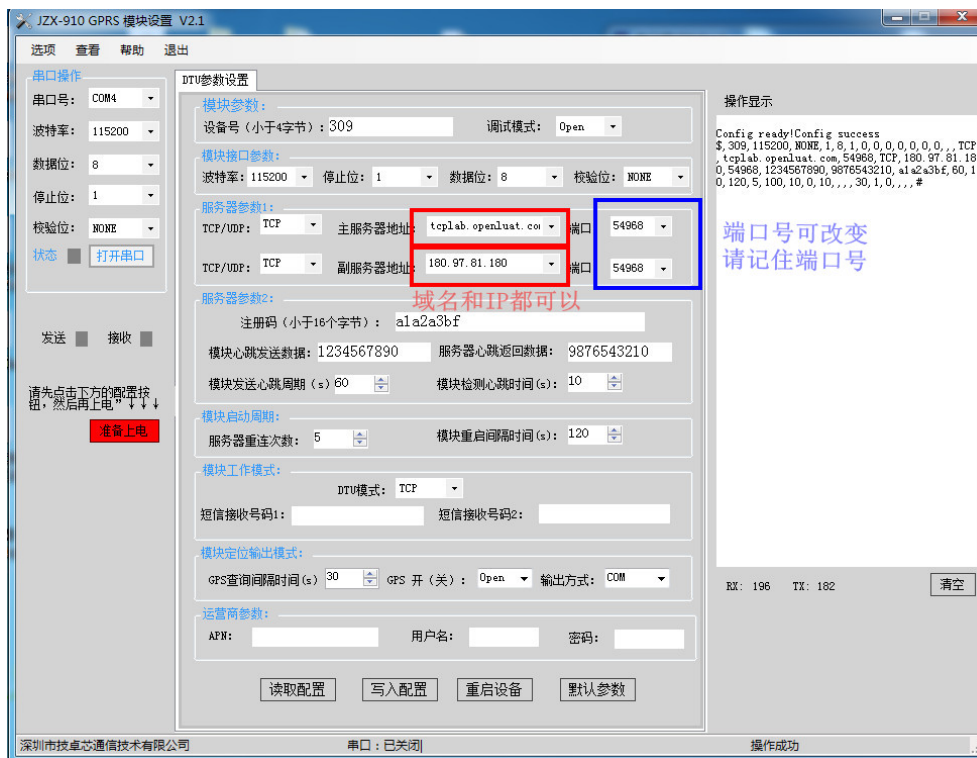
图六 网络平台参数设置
